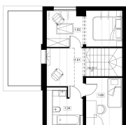
RZUT PARTERU
