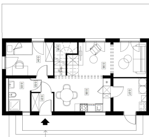
RZUT PARTERU
