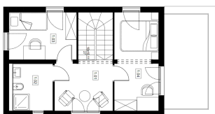
RZUT PIĘTRA
