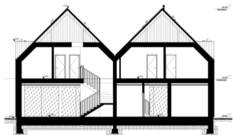
PRZEKRÓJ A-A
