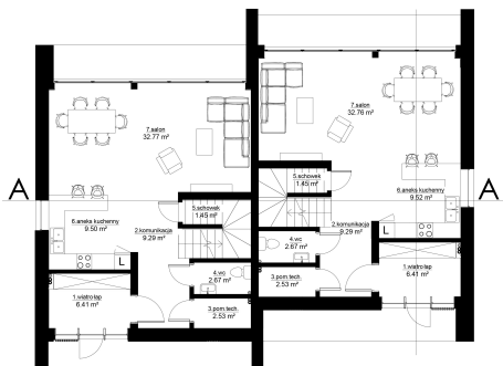
RZUT PARTERU
