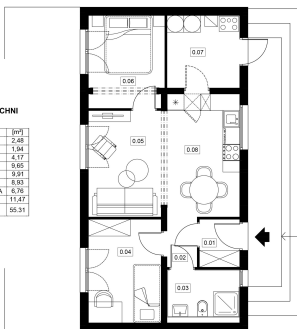
RZUT PARTERU
