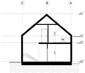
PRZKÓJ A-A
