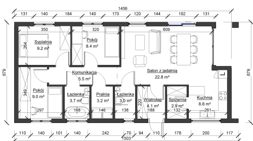
RZUT PARTERU
